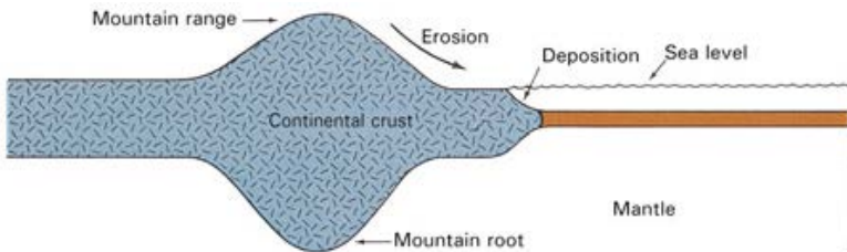
تصویر ۹: تصویر دیگری که نشان می‌دهد کوه‌ها به دلیل ریشه‌های عمیقشان، شکلی میخ ماندگی دارند. ( Earth Science, Tarbuck and Lutgens، ص ۱۵۸ )
