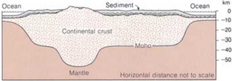
تصویر ۷: کوه‌ها ریشه‌هایی در عمق زمین دارند. ( Earth Press and Siever ص ۴۱۳ )
