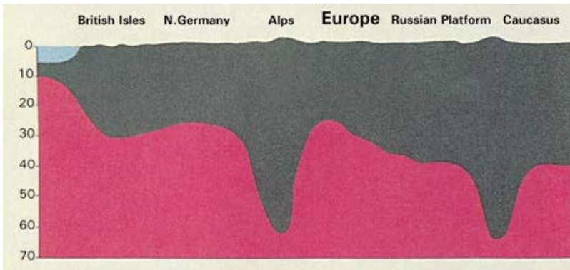
تصویر ۸: نمای کلی نیمرخ. کوه‌ها مانند میخ‌ها، ریشه‌های عمیقی در ژرفای سطح زمین دارند. ( Anatomy of the Earth, Cailleux، ص ۲۲۰ )
